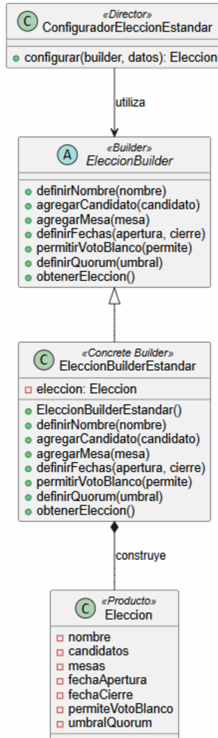
Ilustración 5. Diagrama de clases del patrón Builder aplicado a la configuración de una Elección.
